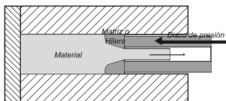
Extrusión inversa
