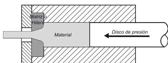
Extrusión directa
